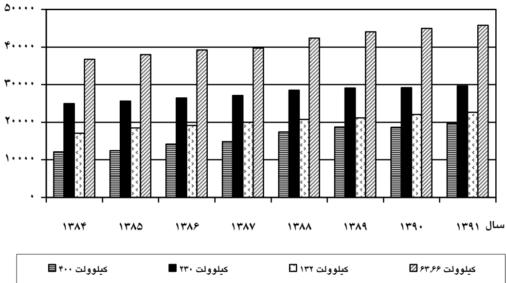
نمودار (۱۹-۱): ظرفیت پست های انتقال و فوق توزیع برق کشور طی سال های ۹۱-۱۳۸۴ (مگاوات آمپر)
